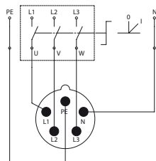
Rozłącznik O-I
