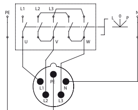
Przełącznik L-O-P
