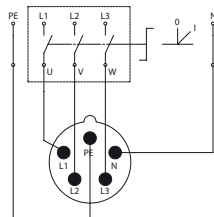
Rozłącznik 0-I
