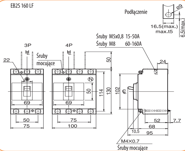
EB2S 160 LF
