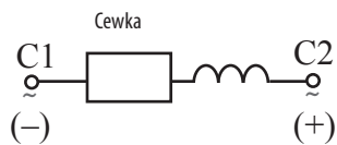
Oznakowanie zacisków styków wyzwalacza wzrostowego
