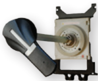
Napęd ręczny RO2...P
