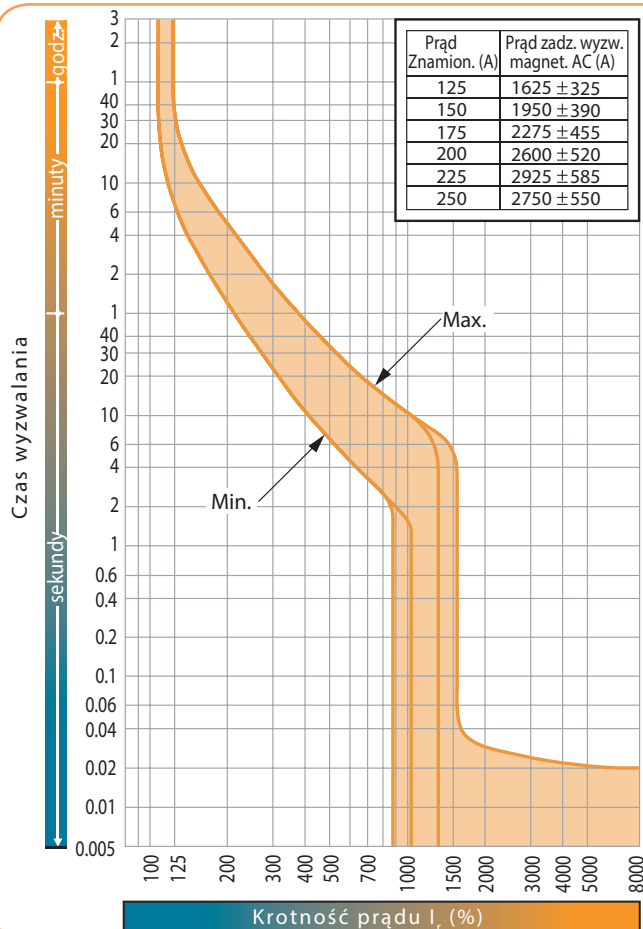
Charakterystyka t-I EB2S 250 LF
