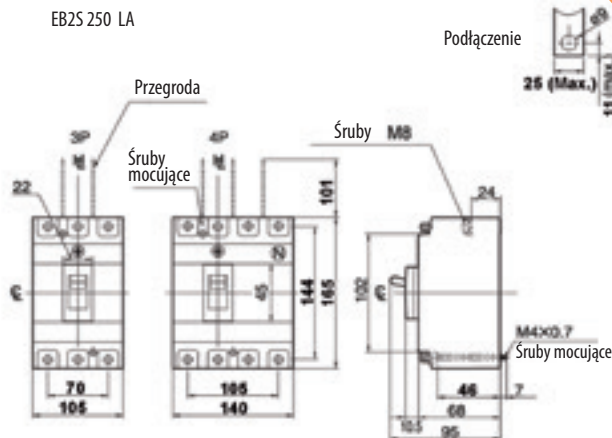
EB2S 250 LA
