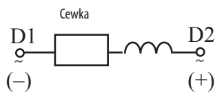
Oznakowanie zacisków styków wyzwalacza podnapięciowego
