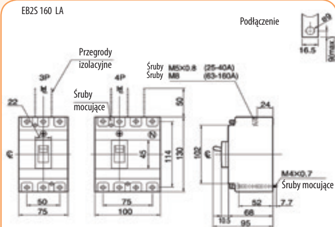
EB2S 160 LA
