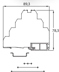
VS 2,5 PE3
