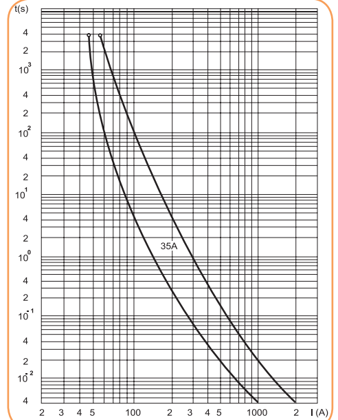
Charakterystyki czasowo-prądowe, pasmowe wkładek topikowych gG (BiWtz) (D) 35A na napięcia 500 i 690 V
