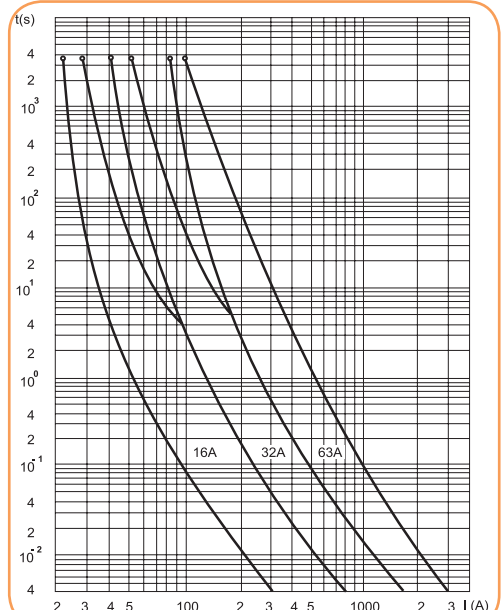
Charakterystyki czasowo-prądowe, pasmowe wkładek topikowych gG (BiWtz) (D) 16, 32, 63A na napięcia 500 i 690 V
