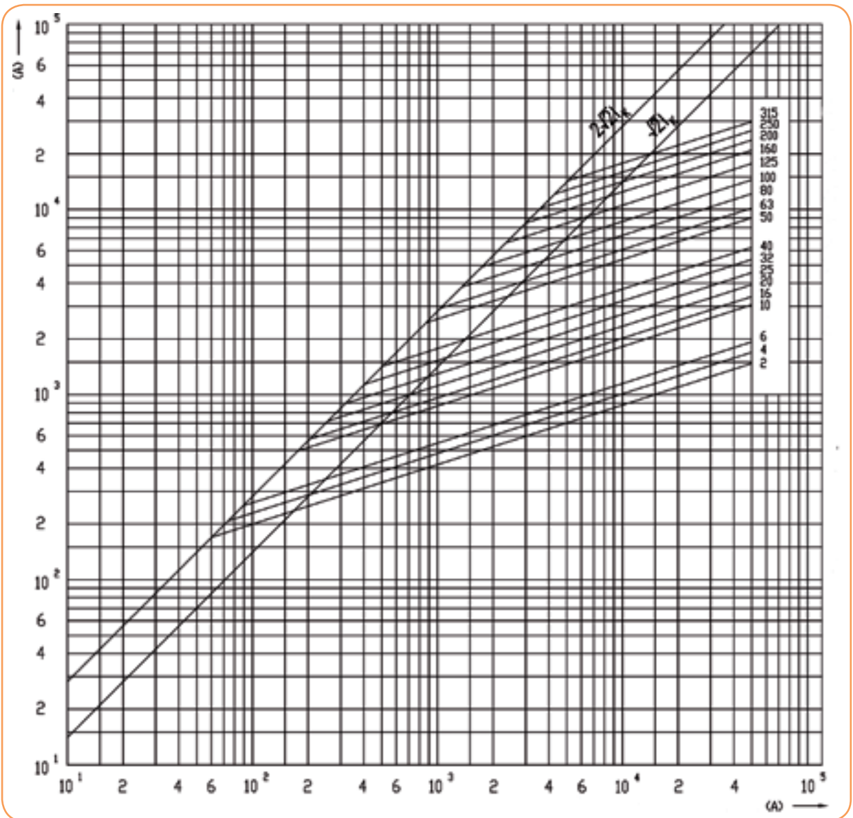
Charakterystyki prądów ograniczonych wkładek VV TERMO VV C, VVT - D, VVT - E
