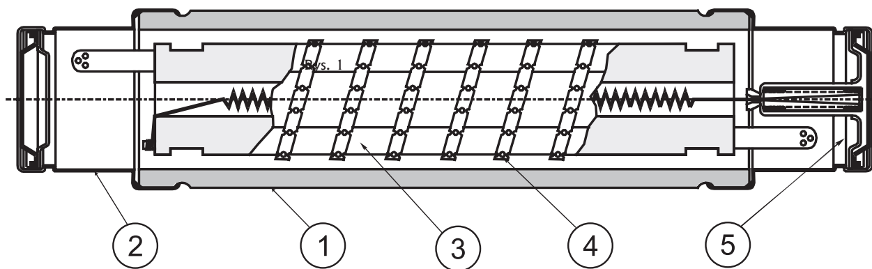
Przekrój podłużny wkładki topikowej VV
