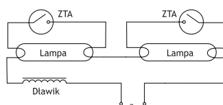
Układ pracy podwójny ZTA 220-240V-
