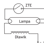
Układ pracy pojedynczy ZTE/2 220-240V-
