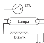
Układ pracy pojedynczy ZTA 110-130V-
