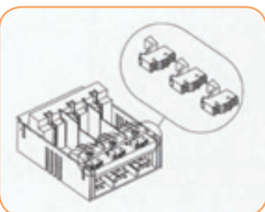
Sposób montażu mikrołączników K-HVL...
