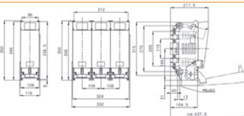
Rysunek wymiarowy rozłączników LTL4A...
