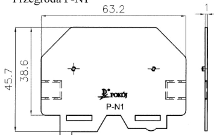
Przegroda P-N1
