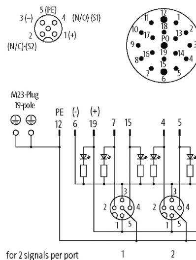
M23-Plug 19-pole
