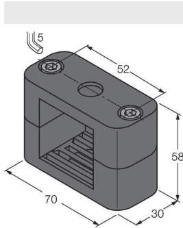
BSS-CP40 6901318 Uchwyt montażowy dla obudów prostokątnych; materiał: Polipropylen
