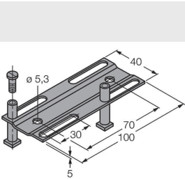
JUSTIERSCHIENE JS 69429 025/037 Szlina montażowa dla obudów prostokątnych CK/CP40; materiał: VA 1.4301
