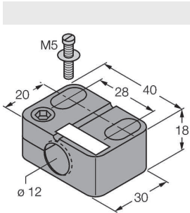
BST-12B 6947212 Klamra montażowa z blokadą dla obudów cylindrycznych, gwintowanych; materiał: PA6
