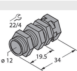
QM-12 6945101 element montażowy szybkiej instalacji z blokadą wysunięcia; materiał: chromowany mosiądz; gwint męski M16 x 1. Uwaga: Zakres detekcji czujników zbliżeniowych może zostać zredukowany, gdy stosowane są elementy montażowe szybkiej instalacji.
