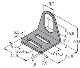
MW-18 6945004 Uchwyt montażowy dla obudów cylindrycznych, gwintowanych; materiał: Stal nierdzewna A2 1.4301 (AISI 304)
