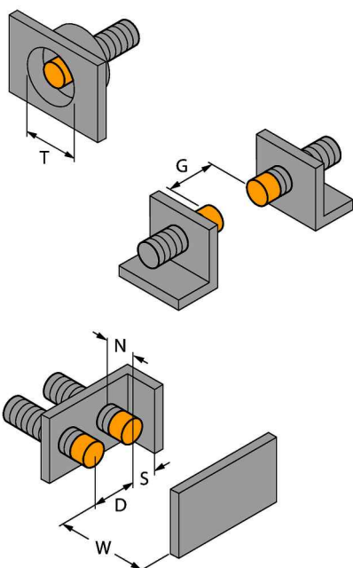
BST-30B 6947216 Klamra montażowa z blokadą dla obudów cylindrycznych, gwintowanych; materiał: PA6
