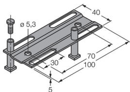
Szyna montażowa dla obudów prostokątnych CK/CP40; materiał: VA 1.4301
