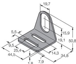
MW-18 6945004 Uchwyt montażowy dla obudów cylindrycznych, gwintowanych; materiał: Stal nierdzewna A2 1.4301 (AISI 304)
