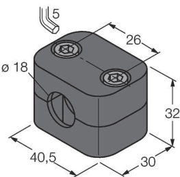
BSS-18 6901320 Uchwyt montażowy dla obudów cylindrycznych, gładkich i gwintowanych; materiał: Polipropylen
