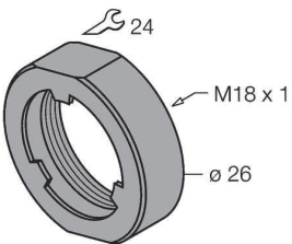
PN-M18 6905310 Nakrętka amortyzująca dla gwintu M18x1; materiał: Stal nierdzewna A2 1.4305 (AISI 303)
