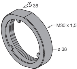
PN-M30 6905308 Nakrętka amortyzująca dla gwintu M30x1; materiał: Stal nierdzewna A2 1.4305 (AISI 303)
