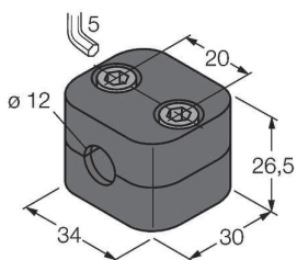
BSS-12 6901321 Uchwyt montażowy dla obudów cylindrycznych, gładkich i gwintowanych; materiał: Polipropylen
