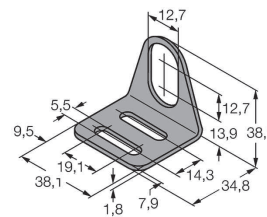
BST-12B 6947212 Klamra montażowa z blokadą dla obudów cylindrycznych, gwintowanych; materiał: PA6
