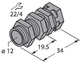
QM-12 6945101 element montażowy szybkiej instalacji z blokadą wysunięcia; materiał: chromowany mosiądz; gwint męski M16 x 1. Uwaga: Zakres detekcji czujników zbliżeniowych może zostać zredukowany, gdy stosowane są elementy montażowe szybkiej instalacji.
