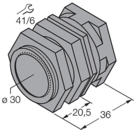
QM-30 6945103 element montażowy szybkiej instalacji z wymuszoną pozycją czujnika; materiał: chromowany mosiądz; gwint męski M36 x 1.5. Uwaga: Zakres detekcji czujników zbliżeniowych może zostać zredukowany, gdy stosowane są elementy montażowe szybkiej instalacji.
