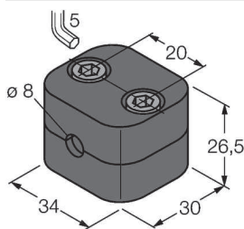
BSS-08 6901322 Uchwyt montażowy dla obudów cylindrycznych, gładkich i gwintowanych; materiał: Polipropylen
