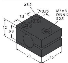
MB580 69479 Uchwyt montażowy dla obudów cylindrycznych, gwintowanych; materiał bloku montażowego: Anodyzowane aluminium
