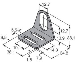
MW-12 6945003 Uchwyt montażowy dla obudów cylindrycznych, gwintowanych; materiał: Stal nierdzewna A2 1.4301 (AISI 304)
