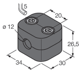
MW-12 6945003 Uchwyt montażowy dla obudów cylindrycznych, gwintowanych; materiał: Stal nierdzewna A2 1.4301 (AISI 304)
