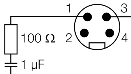
Schemat podłączenia
