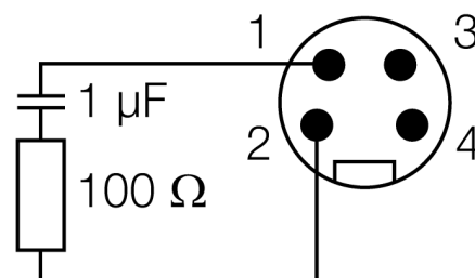
Schemat podłączenia
