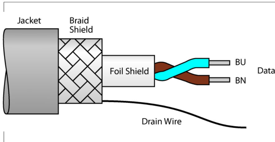
Przekrój poprzeczny przewodu
