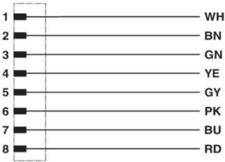
Cable
