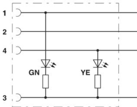
Cable
