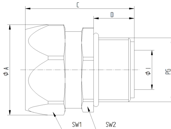
SILVYN HIPROJACKET AMG PG
