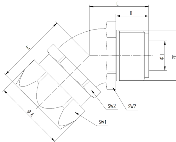
SILVYN HIPROJACKET AMG 45° PG
