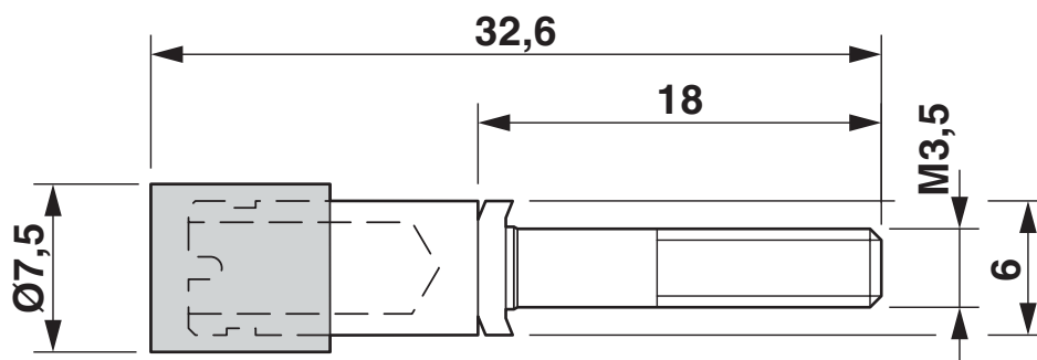
Rysunek wymiarowy
