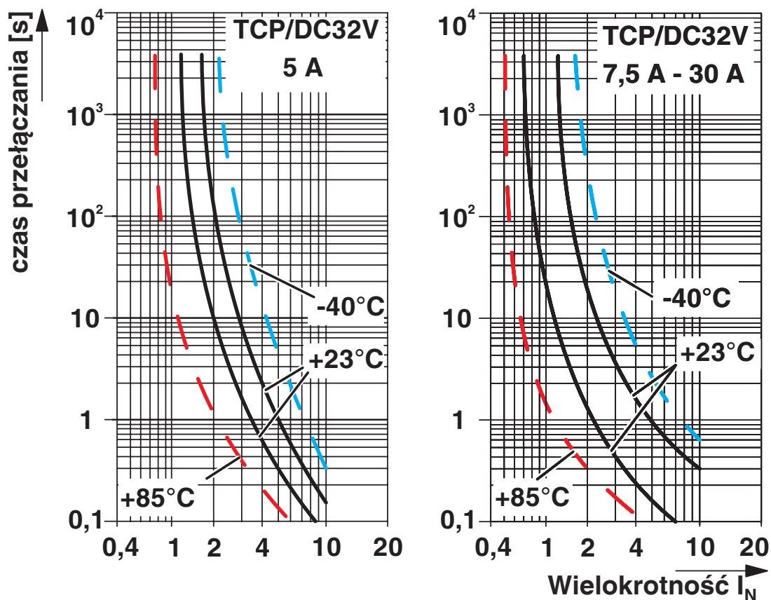
Charakterystyka wyzwalania
