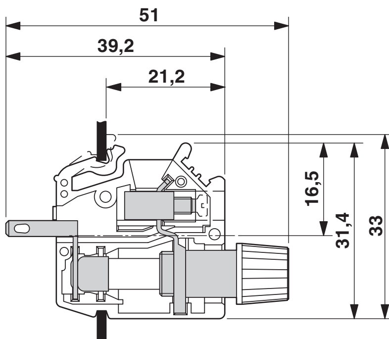
Rysunek wymiarowy
