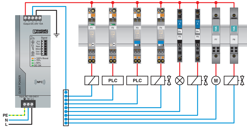
rysunek aplikacji
