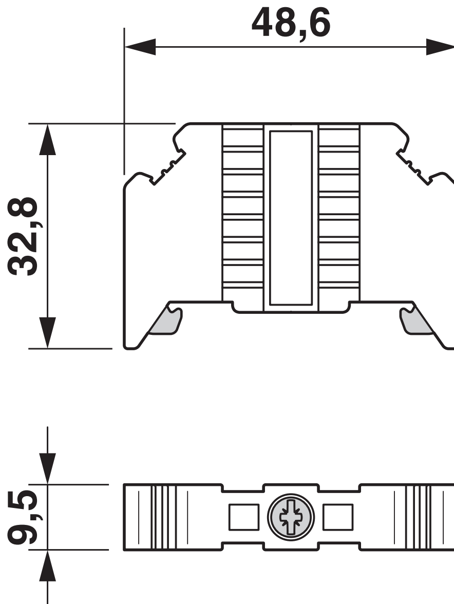
Rysunek wymiarowy
