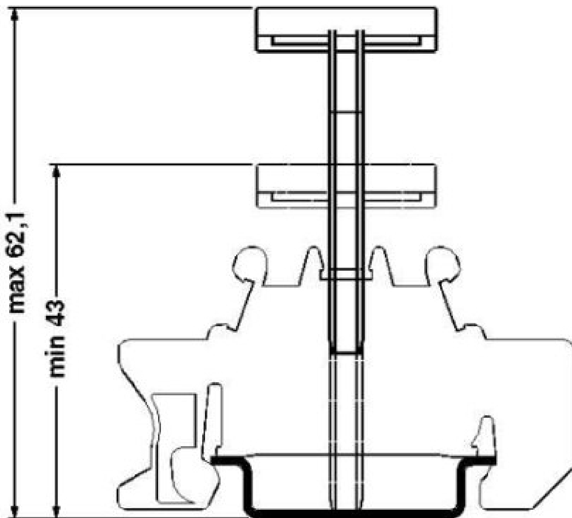
Rysunek wymiarowy
