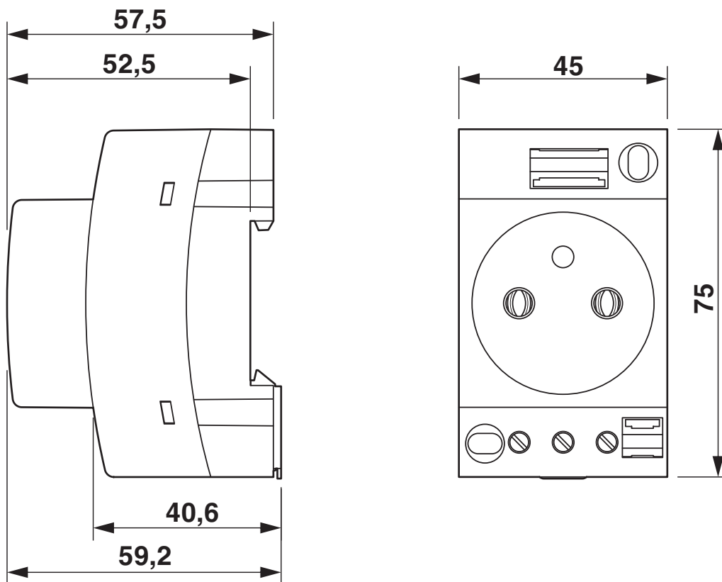
Rysunek wymiarowy
