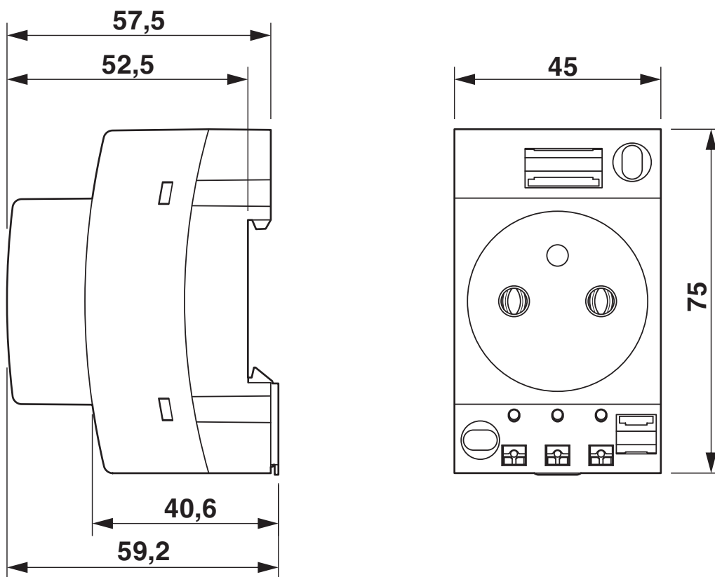
Rysunek wymiarowy
