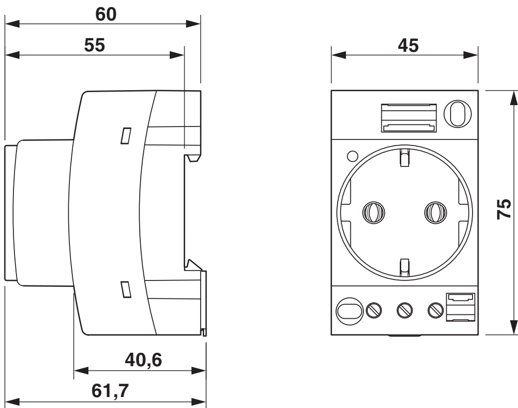
Rysunek wymiarowy
