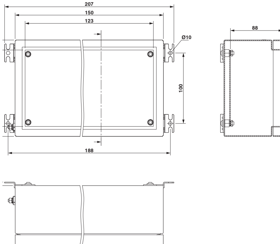
Rysunek wymiarowy
