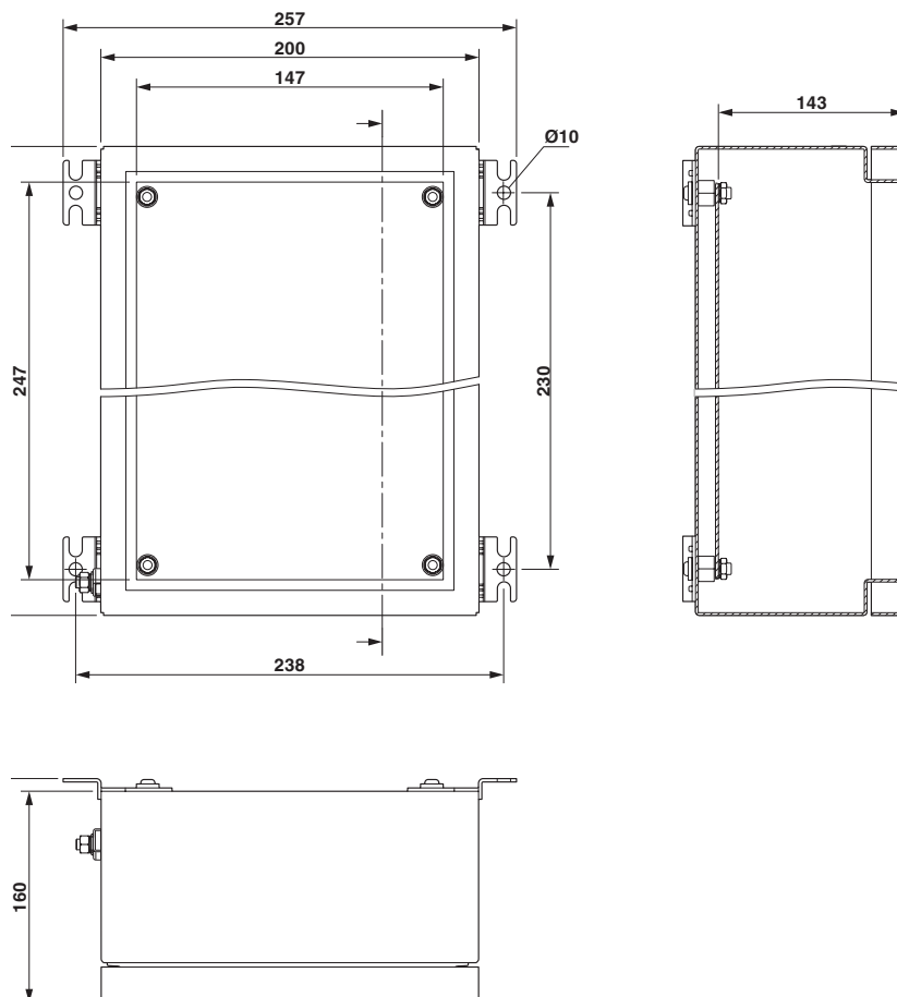
Rysunek wymiarowy
