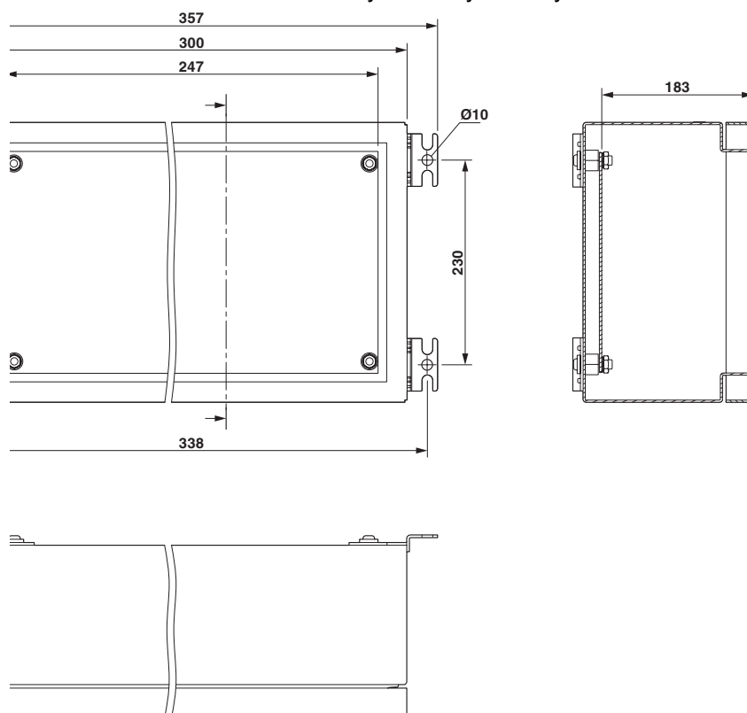
Rysunek wymiarowy
