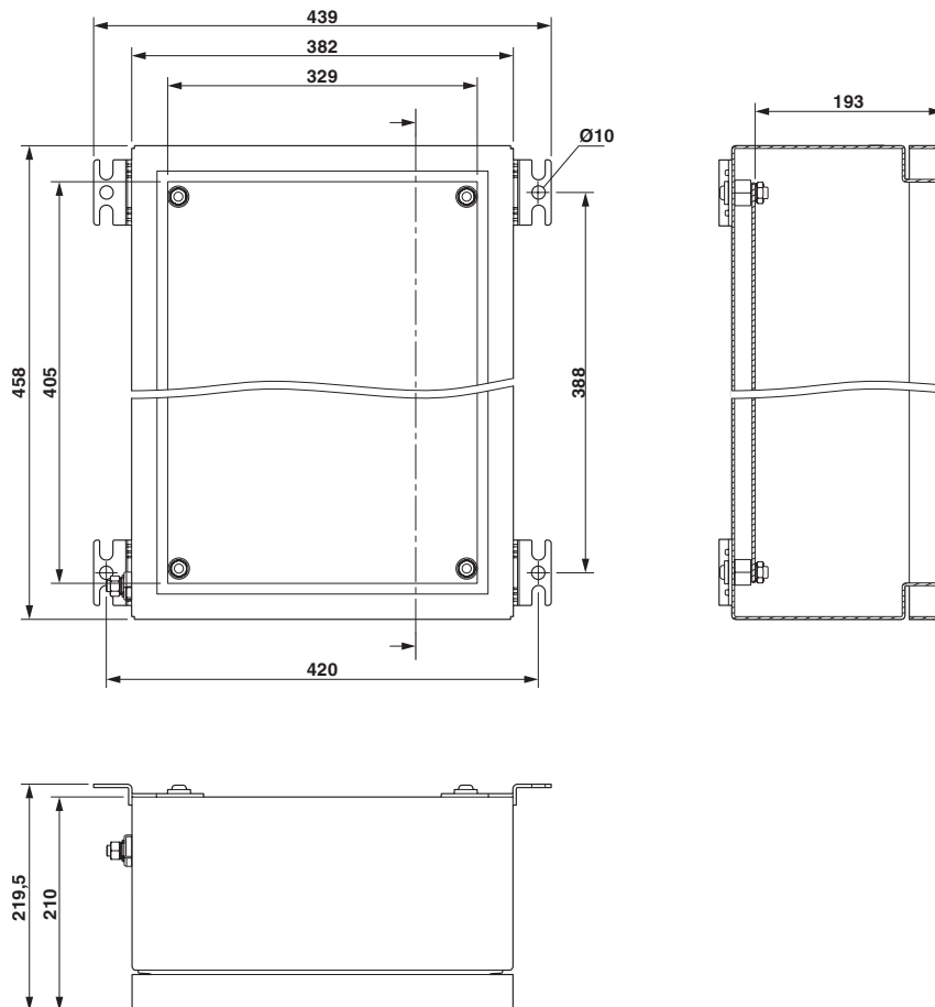
Rysunek wymiarowy
