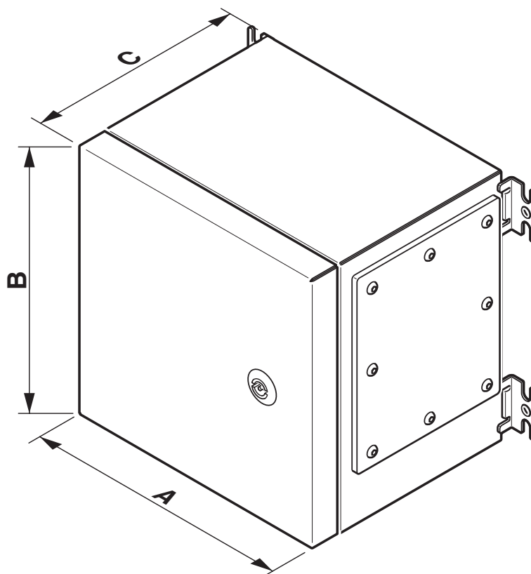
Rysunek schematyczny
