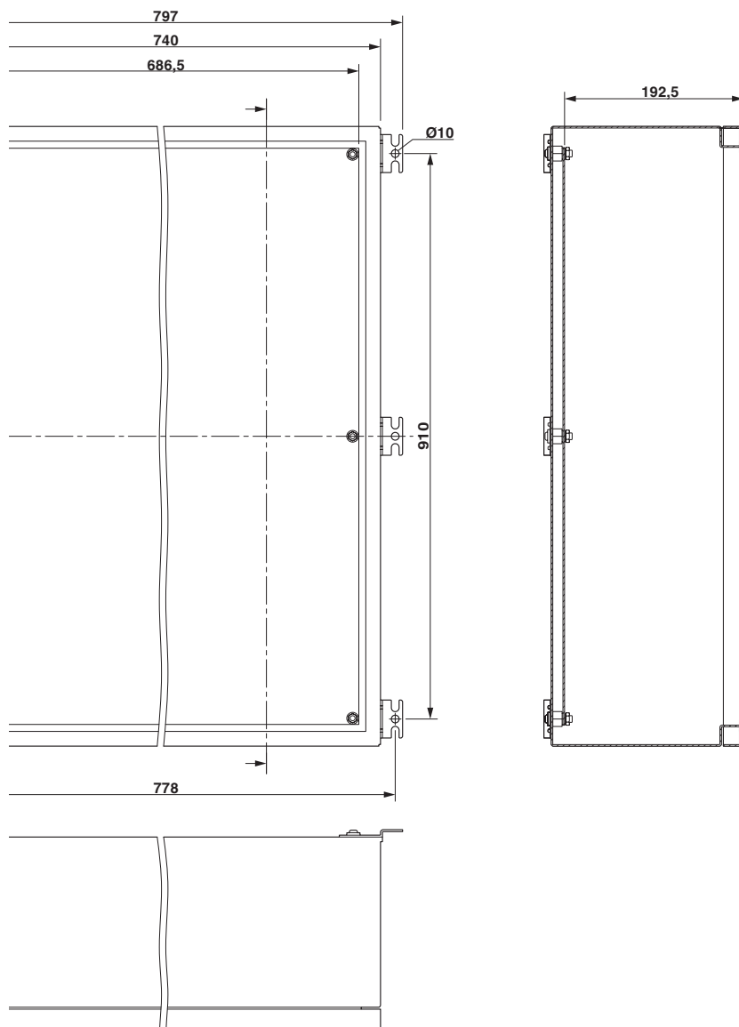
Rysunek wymiarowy
