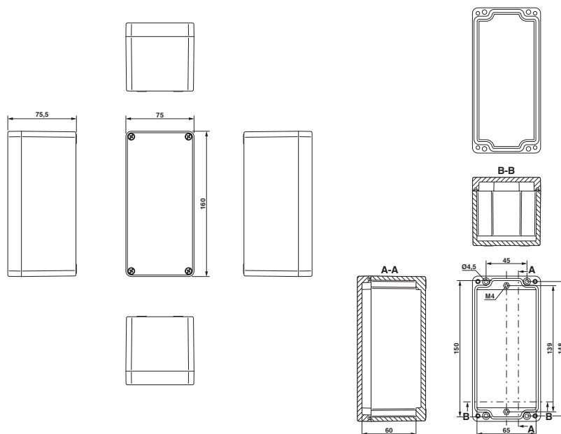
Rysunek wymiarowy
