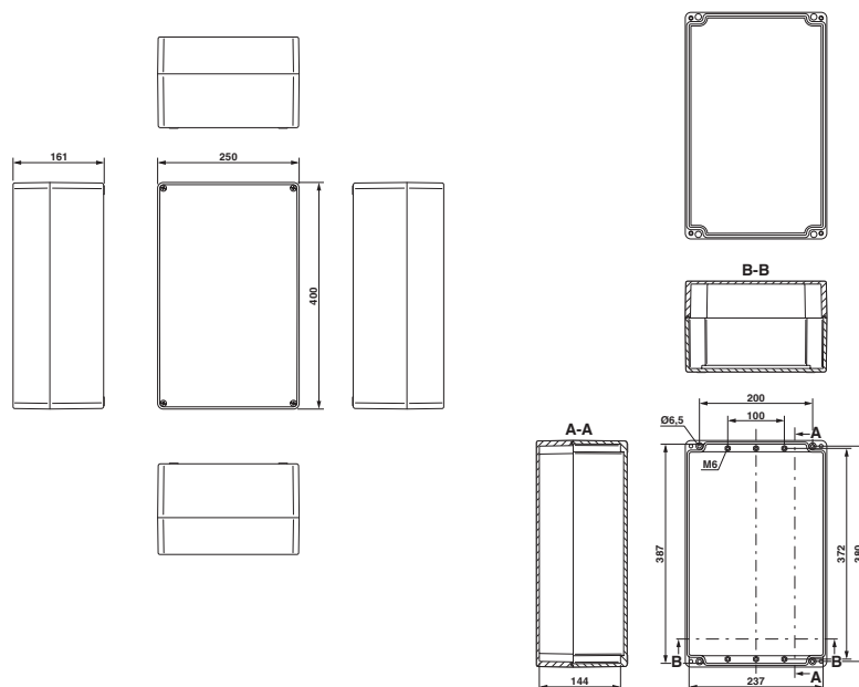
Rysunek wymiarowy
