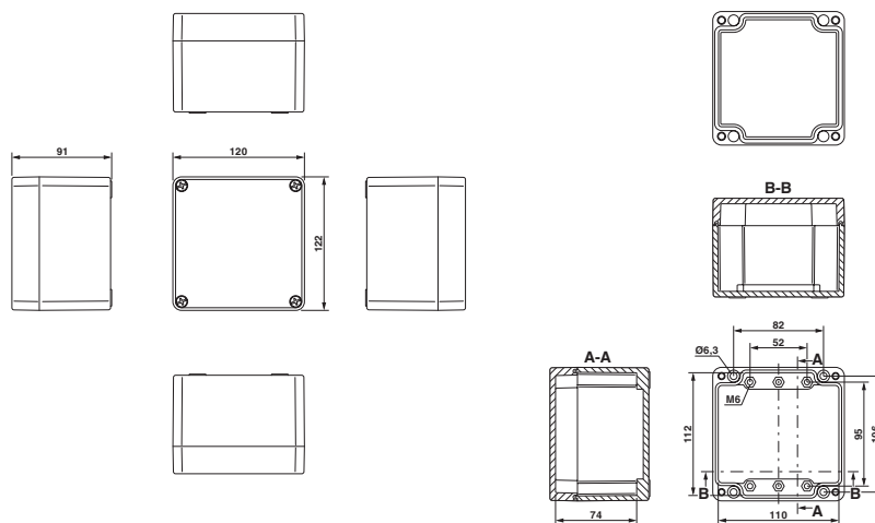
Rysunek wymiarowy
