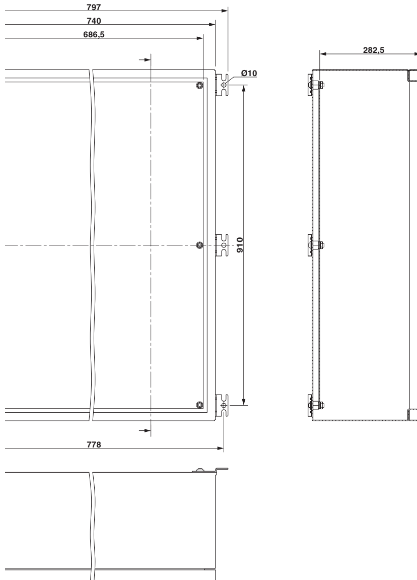
Rysunek wymiarowy
