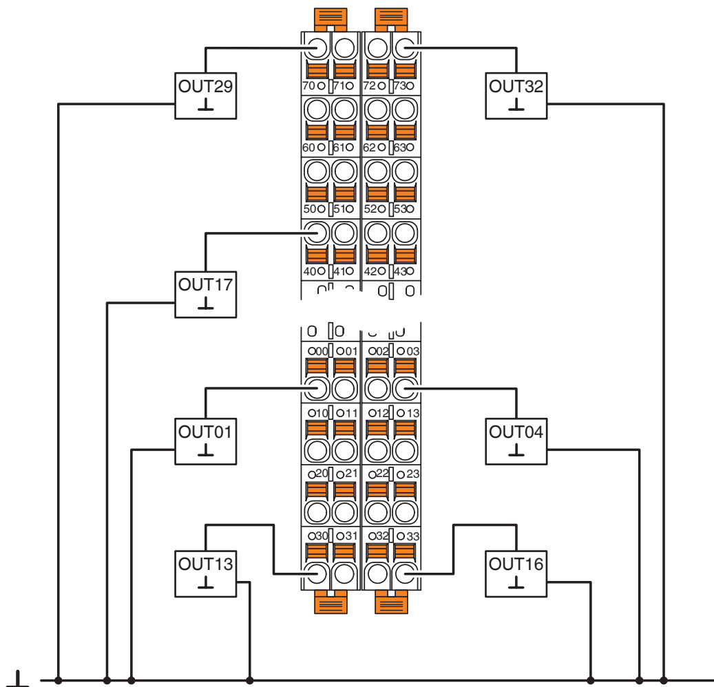
rysunek złączy
