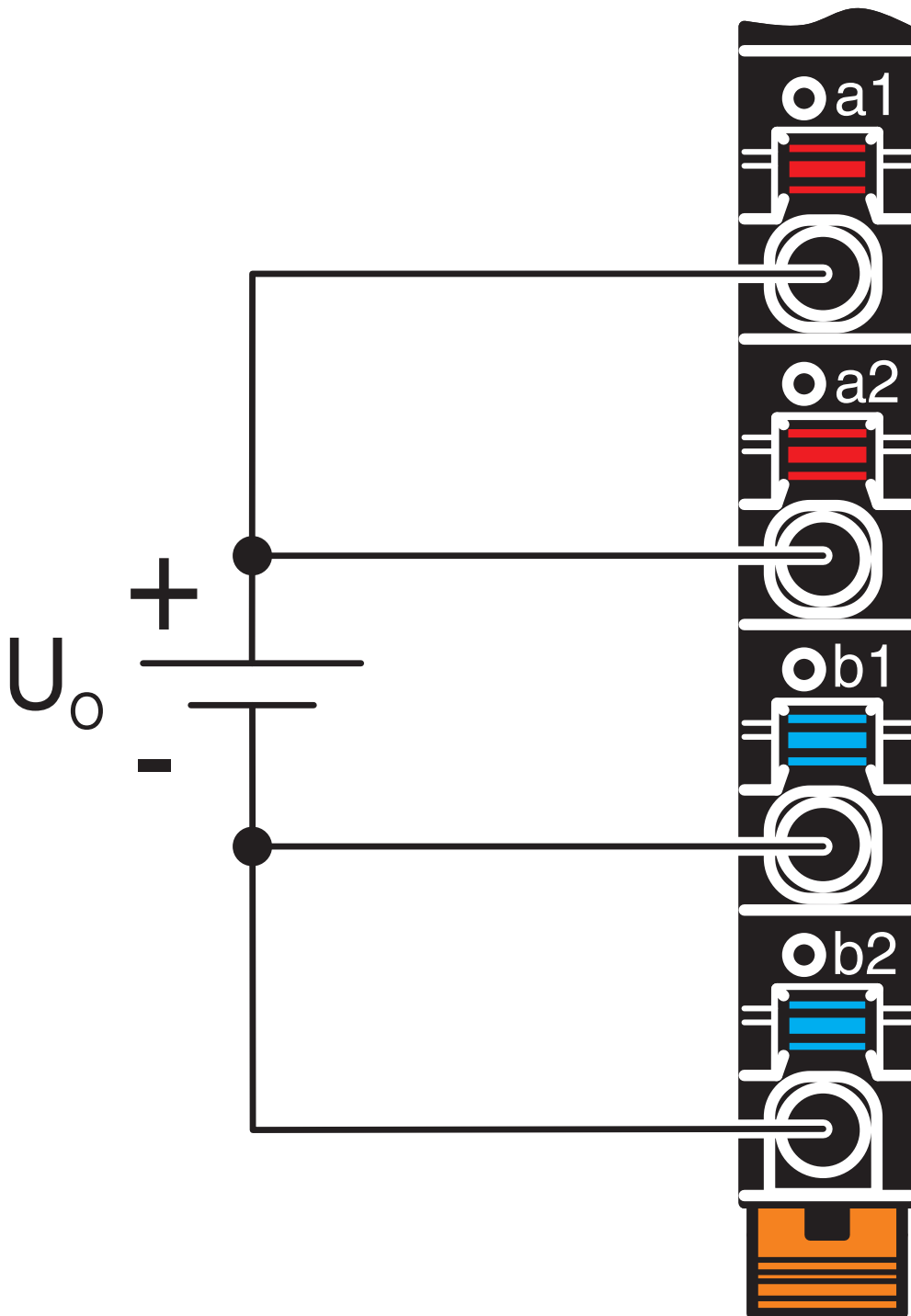
rysunek złączy
