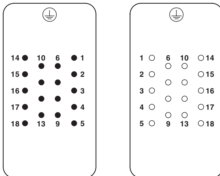
Rysunek schematyczny
