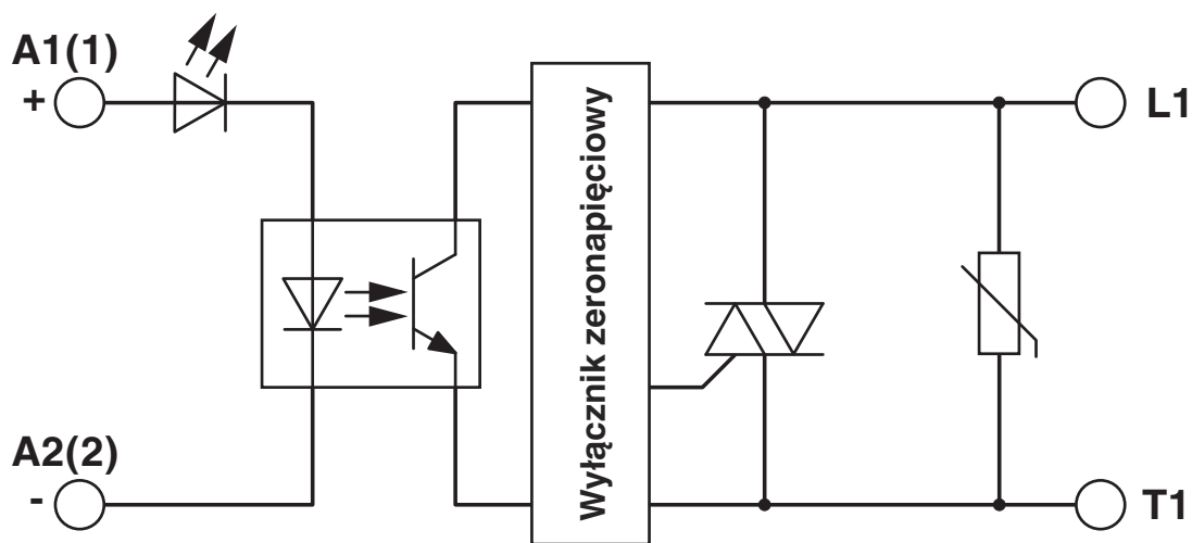
Schemat blokowy
