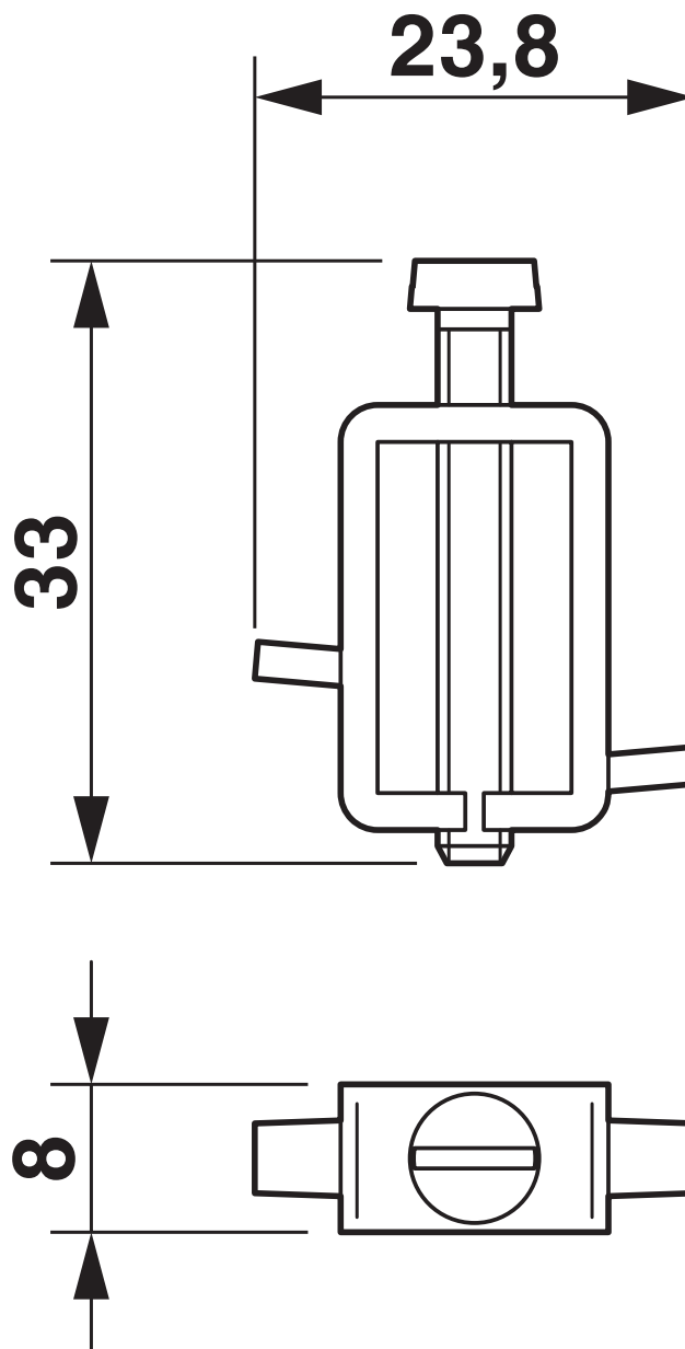
Rysunek wymiarowy
